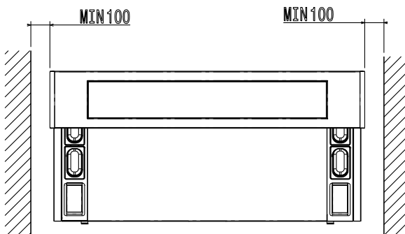
Boven aanzicht
